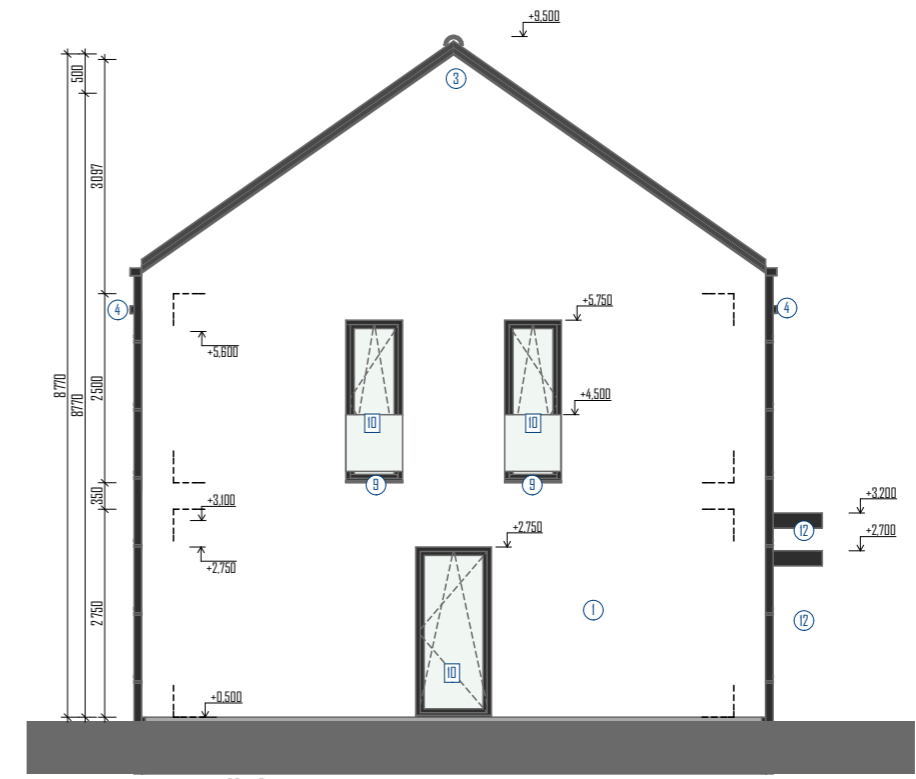
SO-101_POHLED JIŽNÍ
